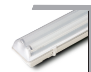
Model : PEL 120 NM/SL Lamp Type : 1 x 18/20W FTL Accumulator : SLA Battery Backup : 1 Hrs. Standard Pkg.: 2 pcs. Box size in mm : 310x160x700
